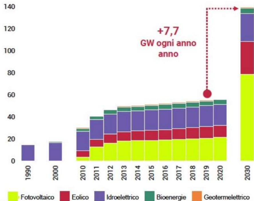
Potenza installata di fonti rinnovabili in Italia – Roadmap I4C (milioni di kW)
